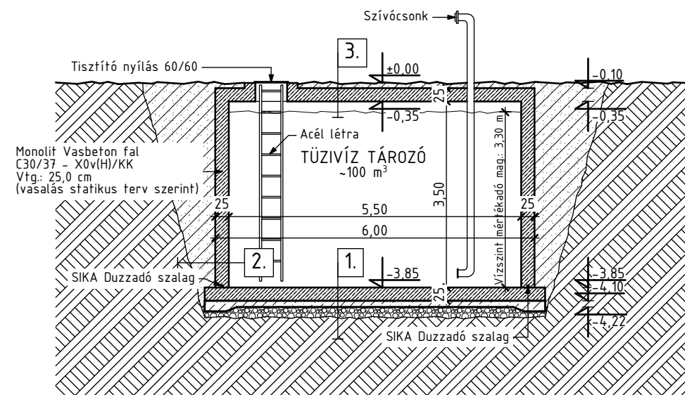
A-A Metszet M 1:100
