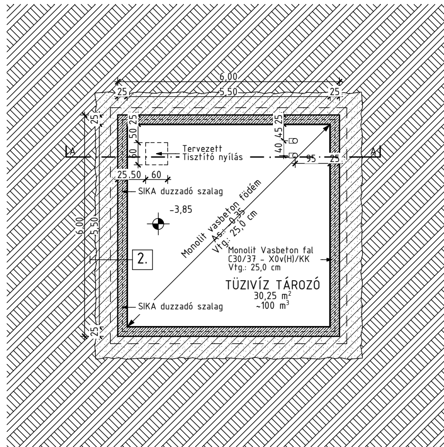
Alaprajz M 1:100
